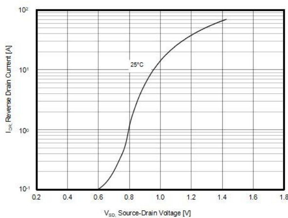
Figure5. Source-Drain Diode Forward Volt
