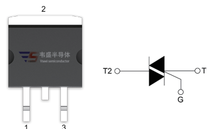
TO-263
