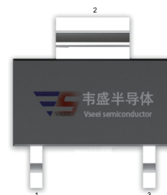
SOT-223-2
