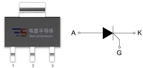
SOT-223
