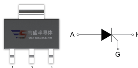
SOT-223
