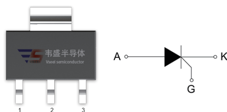
SOT-223
