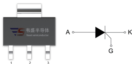
SOT-223
