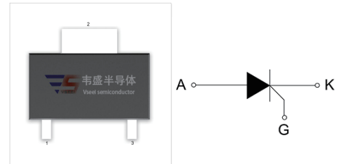
SOT-89-2
