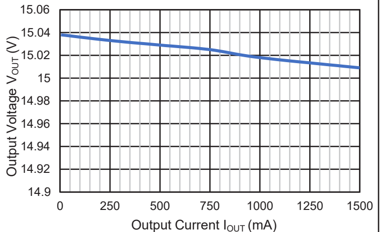
VS7815E Load Regulation
