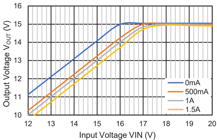
VS7815E Dropout Voltage
