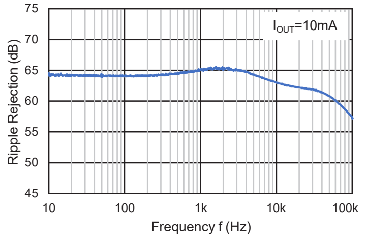
VS7815E Ripple Rejection
